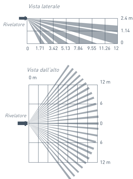
FIGURA 3. Zone di rilevazione del rivelatore
